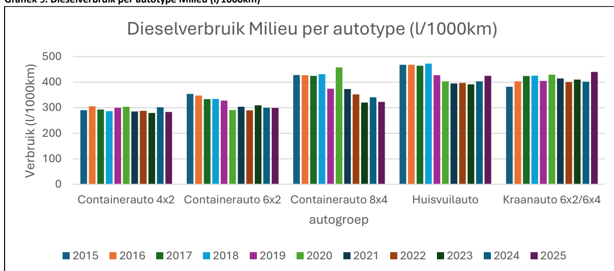
Grafiek 9. Diesilverbruik per autotype Milieu (l/1000km)
