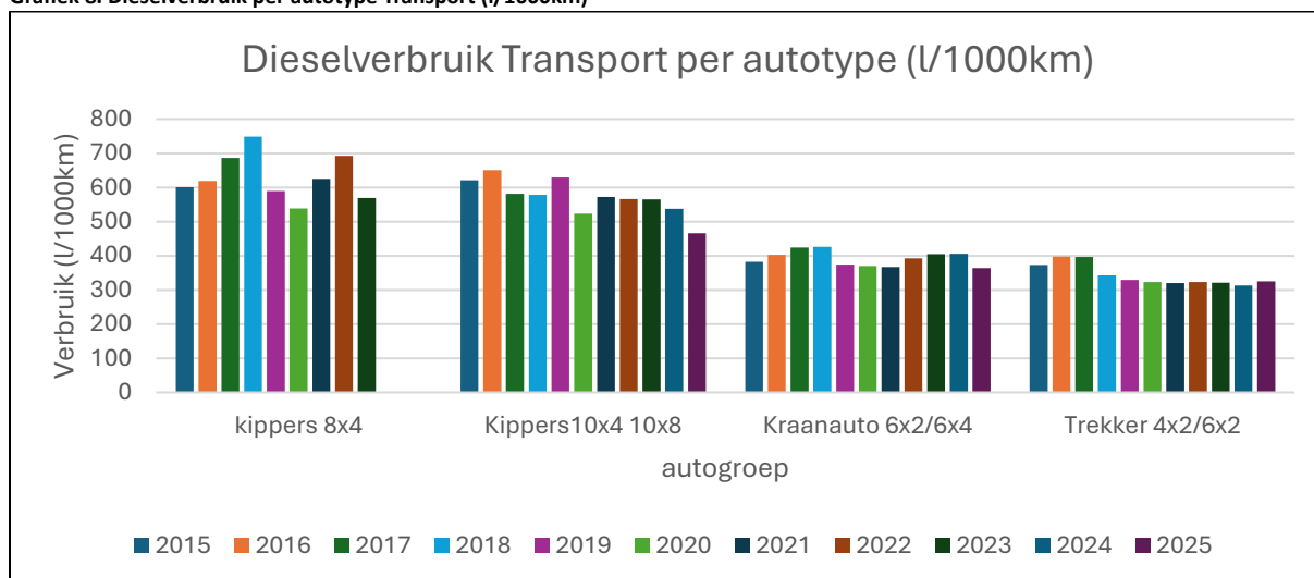
Grafiek 8. Diesilverbruik per autotype Transport (l/1000km)
