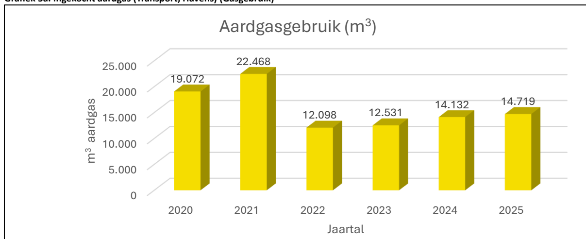
Grafiek 5a. Ingekocht aardgas (Transport, Havens) (Gasgebruik)
