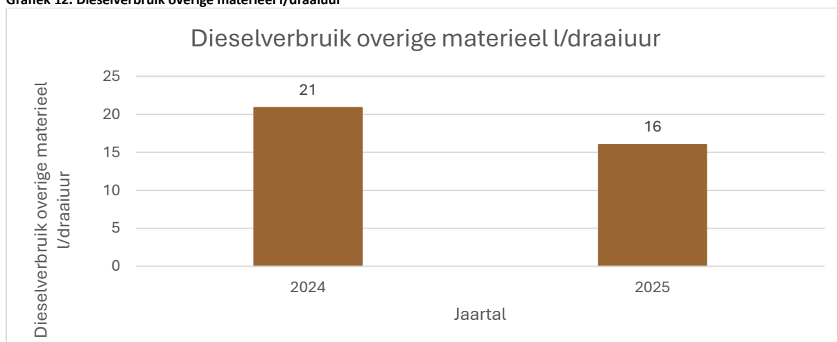
Grafiek 12. Diesilverbruik overige materieel l/draaiuur
